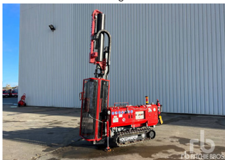
2019 Socomafor 10
